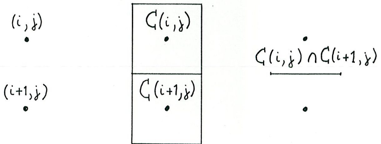
FIGURE 1. C(i, j) \cap C(i+1, j) \neq \emptyset .
